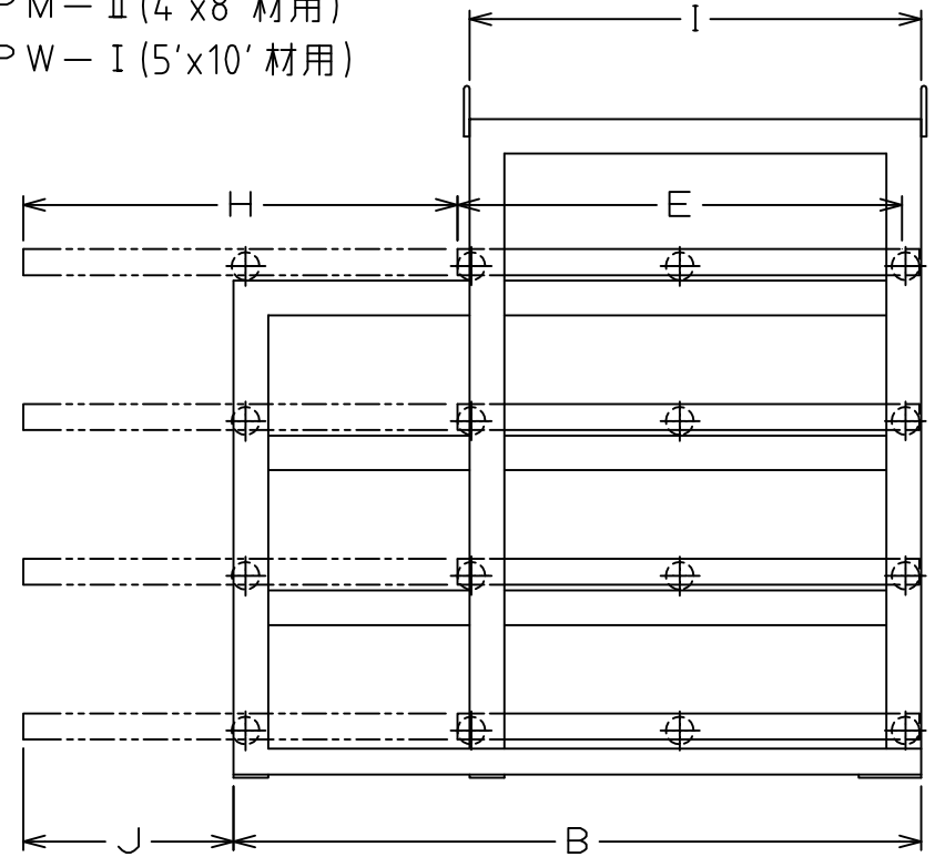
スライダー Pシリーズ 五段タイプ 寸法表
